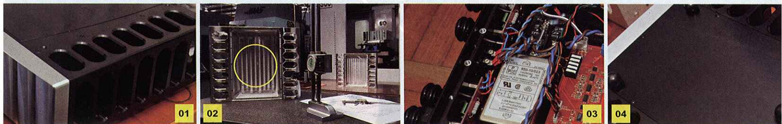
01 機身設計已經是一個大型散熱器。 02 機殼由整件鋁金屬以電腦車床製作，供電與放大電路之間只有一個小孔。 03 內置EMI Filter，可隔絕由電源傳入的外來干擾。 04 機腳採用球形設計，減少接觸面。
