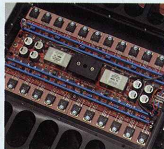
● 放大線路由多顆晶體管所組成。
